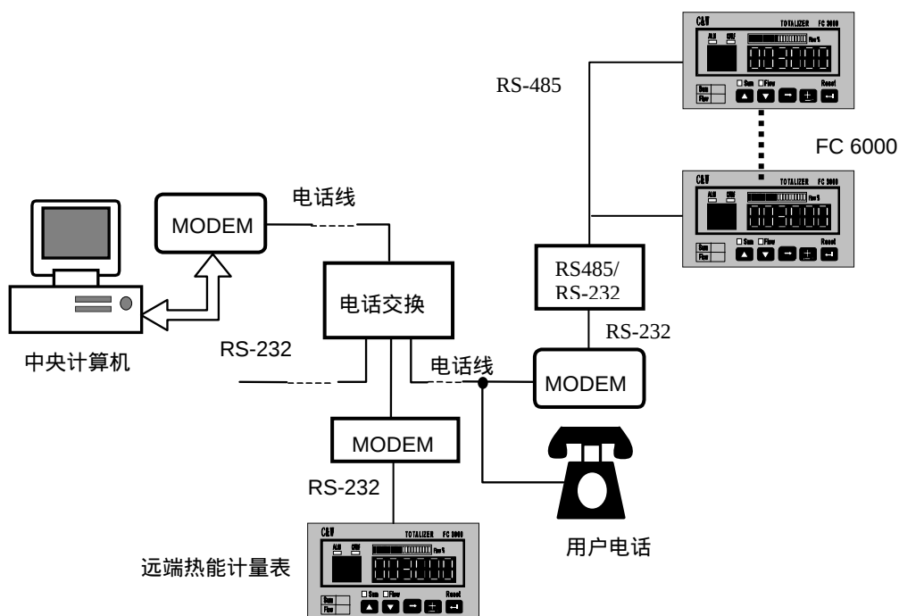
图 计算机远程抄表系统图
