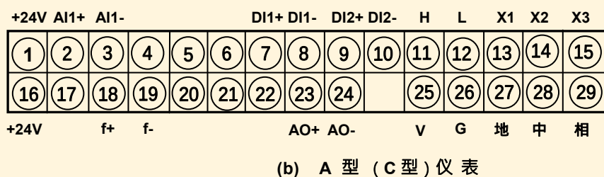
图 2 线路连接与流量转换器端子排列
