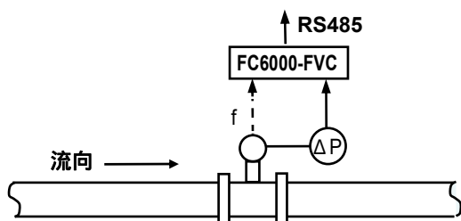
图1 FVC质量流量计系统图
