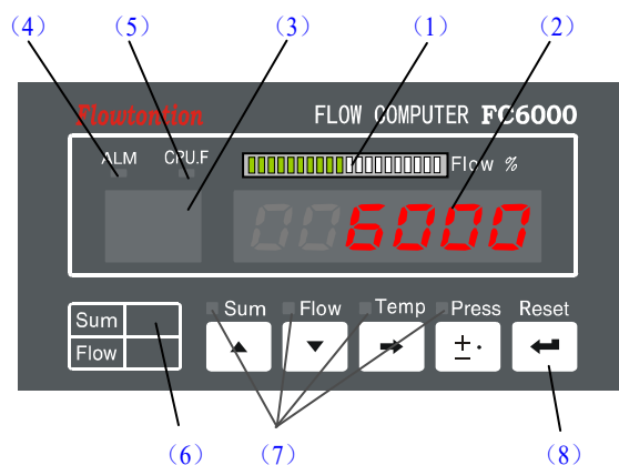
图 7 流量显示装置面板示意
