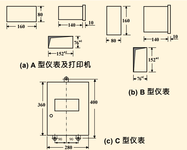
图 4 显示仪外形尺寸及开孔尺寸
